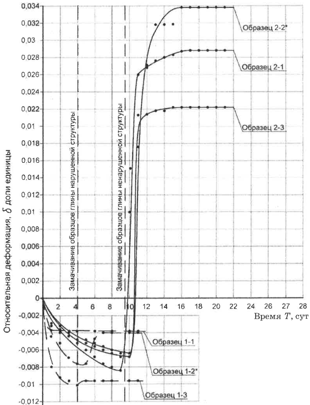
Рис. 2. График осадки и набухания образцов глины нарушенной и ненарушенной структуры под нагрузкой 0,018 МПа в компрессионном приборе: сплошные линии – образцы ненарушенной структуры; штриховые линии – образцы нарушенной структуры
