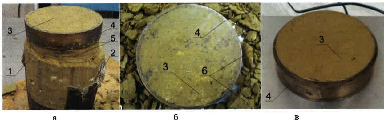
Рис. 1. Вырезание из монолита кольцом компрессионного прибора образца глины ненарушенной структуры (а), вид этого образца в кольце (б) и вид образца глины нарушенной структуры, вырезанного кольцом из монолита, сформированного уплотнением грунта валовой пробы в приборе стандартного уплотнения (в): 1 – монолит; 2 – упаковка; 3 – образец; 4 – кольцо компрессионного прибора; 5 – тонкие прослои и линзы алевритов; 6 – куски глины, срезанные с монолита в процессе вырезания образца
