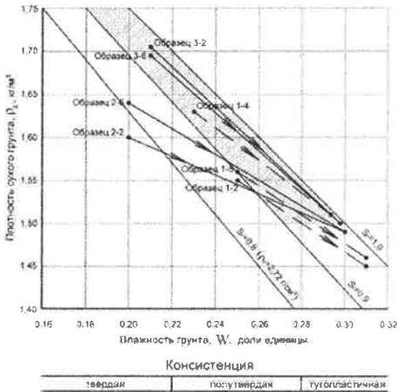
Рис. 3. Изменение плотности и влажности глины при свободном набухании (а) и при набухании под нагрузкой 0,018 МПа (б): сплошные линии – образцы ненарушенной структуры; штриховые линии – образцы нарушенной структуры. Номера образцов показаны у точек, характеризующих их начальную плотность-влажность; заштрихована зона требуемых значений плотности-влажности грунта; начальные значения плотности-влажности образцов 1-1, 1-2*
