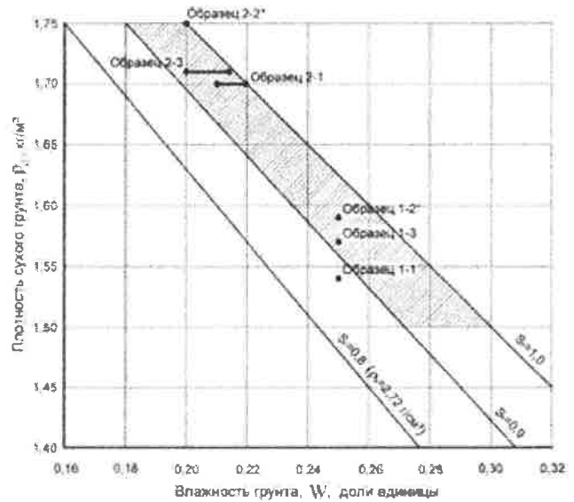
Рис. 3. Изменение плотности и влажности глины при свободном набухании (а) и при набухании под нагрузкой 0,018 МПа (б): сплошные линии – образцы ненарушенной структуры; штриховые линии – образцы нарушенной структуры. Номера образцов показаны у точек, характеризующих их начальную плотность-влажность; заштрихована зона требуемых значений плотности-влажности грунта; начальные значения плотности-влажности образцов 1-1, 1-2*
